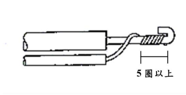
圖二四~一○ 不同線徑之單線終端連接法
